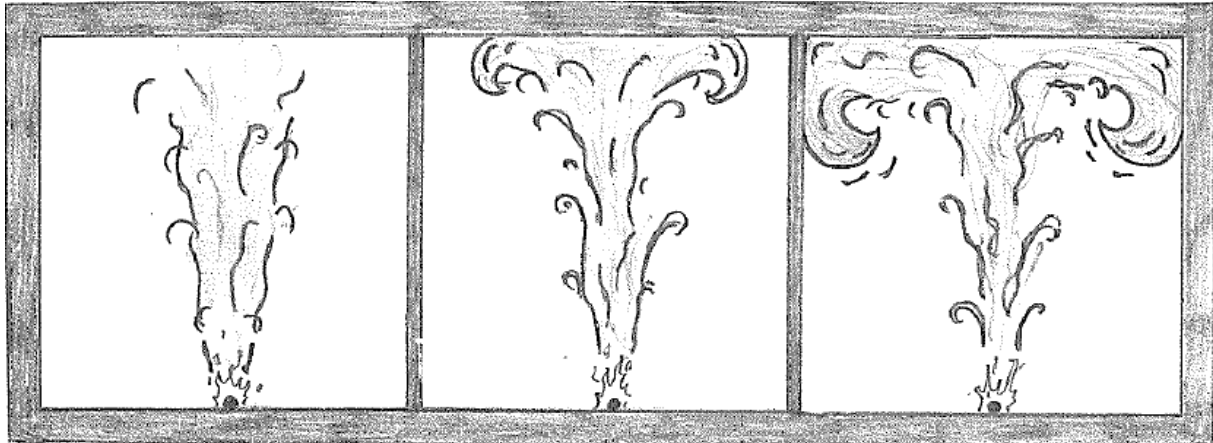
Figur 4 – Dannelsen av røyklag. Bildet til venstre: røyksoyle er dannet. Bildet i midten: Røyksoyle treffer taket og danner en takjet. Bildet til høyre: Røyk avbøyes ved veggene.
