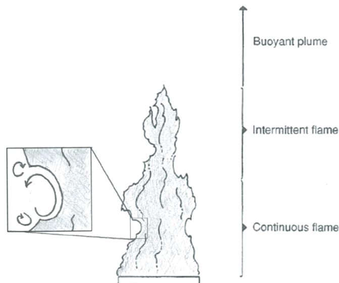
Figur 8 – McCaffreys inndeling av røyksøylen med utdrag av turbulent virvel (Karlsson & Quintiere, 2000)
