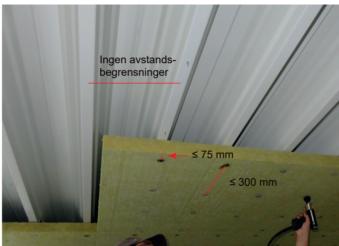
Viser ferdig brannbeskyttelse av trapesformet metallplater med isolasjon, dimensjon 1000x1200mm Isover FireProtect 150 plate markert med rød linje og viser maksimal avstand for sveisepinnene.
