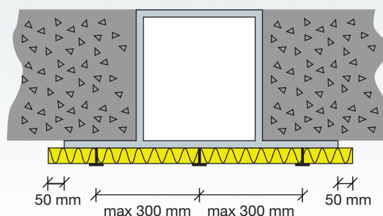
Med isolering av kanten på underflens
